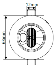
Obr. 2 Rozměry - čelní pohled
