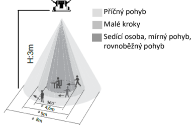
Obr. 6 Pohled zezadu
