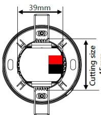
Obr. 4 Rozměry - pohled zezadu
